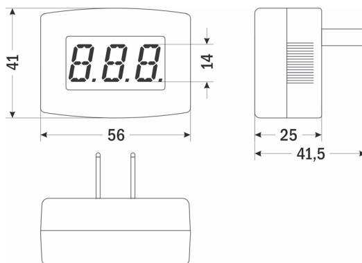
Рис. 3 – Размеры прибора
